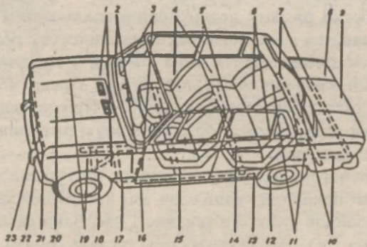
Зоны антикоррозионной обработки кузова автомобиля Ваз:
