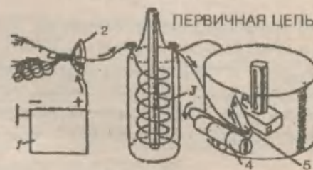
1. Аккумуляторная батарея. 2. Выключатель зажигания. 3. Первичная обмотка катушки зажигания. 4. Конденсатор. 5. Контакт прерывателя-распределителя.
