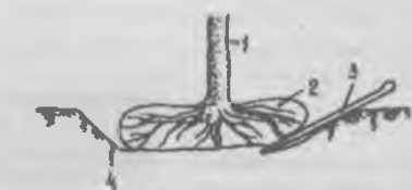
Рис. 1. Схема подрезки кома земли при выемке дерева
