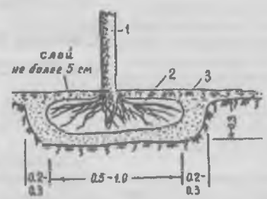
Рис. 3. Схема посадки дерева
