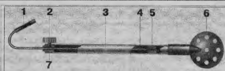
Устройство «черпагорика»: 1 — предохранительная трубка; 2 — винт; 3 — алюминиевая трубка; 4 — шток; 5 — поршень; 6 — черпак; 7 — втулка.
