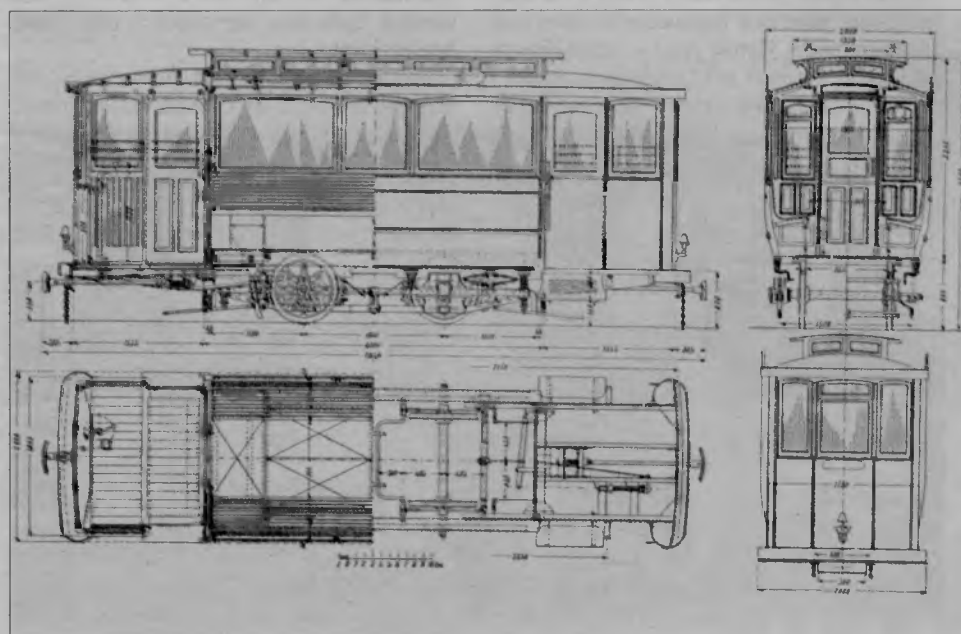
Чертеж вагона мурманского трамвая.
