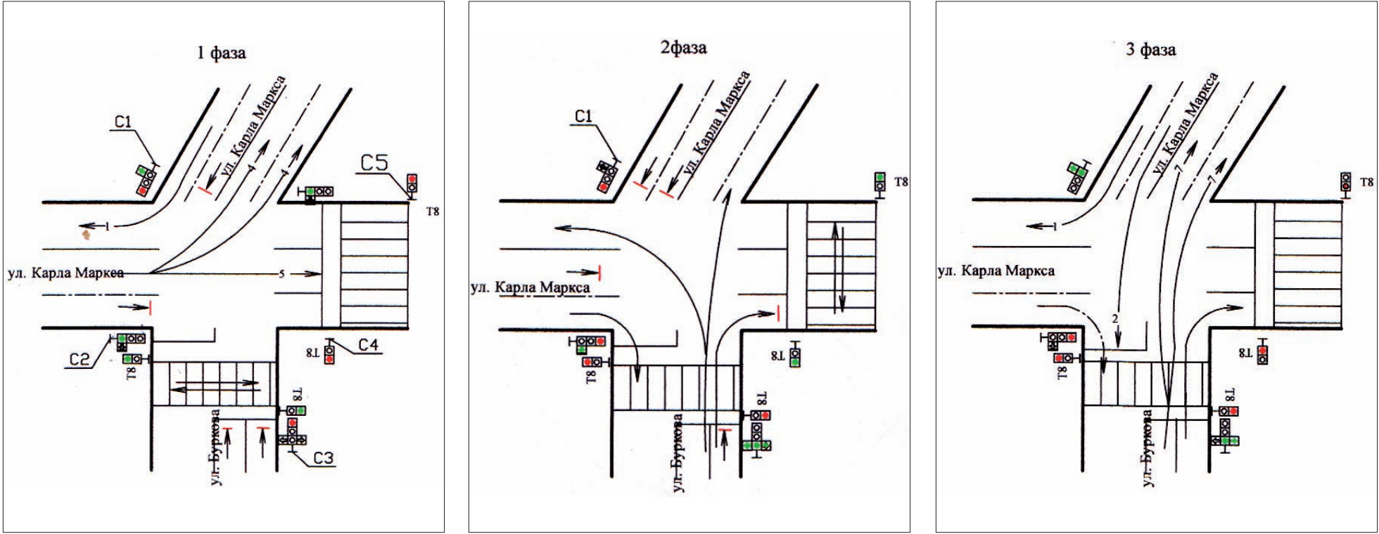
Схема пофазного разъезда на пересечении улиц Карла Маркса и Буркова
