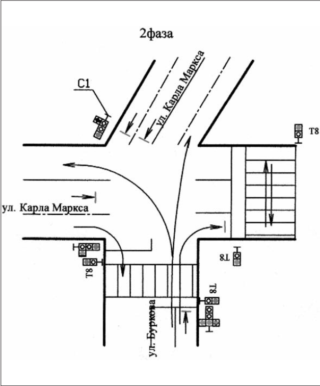
Схема пофазного разъезда на пересечении улиц Карла Маркса и Буркова
