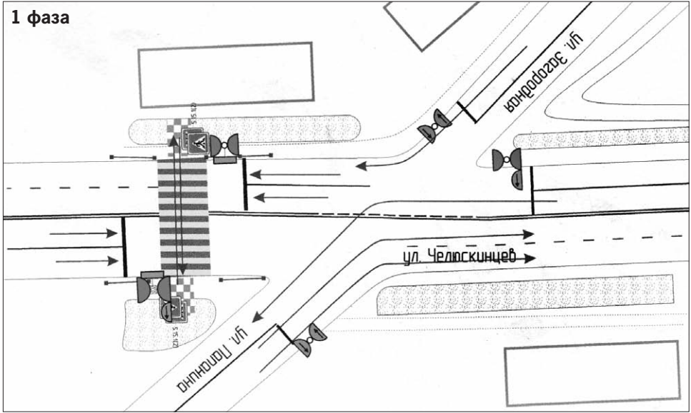
Схема пофазного разъезда на пересечении улиц Папанина и Челюскинцев
