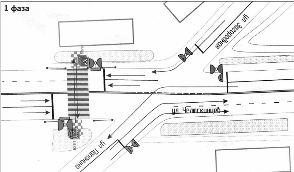
Схема пофазного разъезда на пересечении улиц Папанина и Челюскинцев
