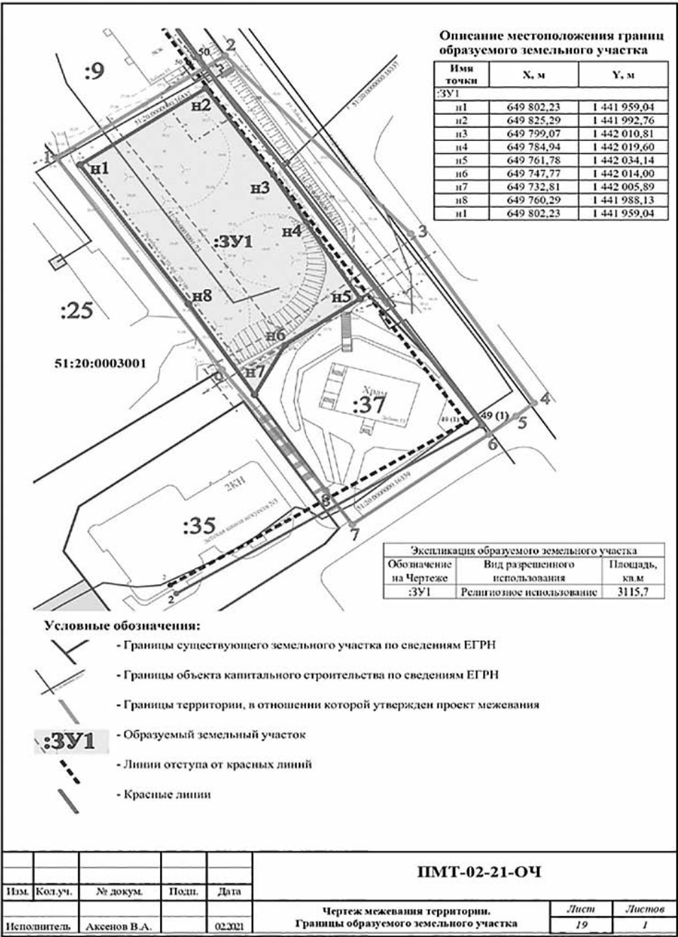
2.3. Чертеж межевания территории. Границы образуемого земельного участка
