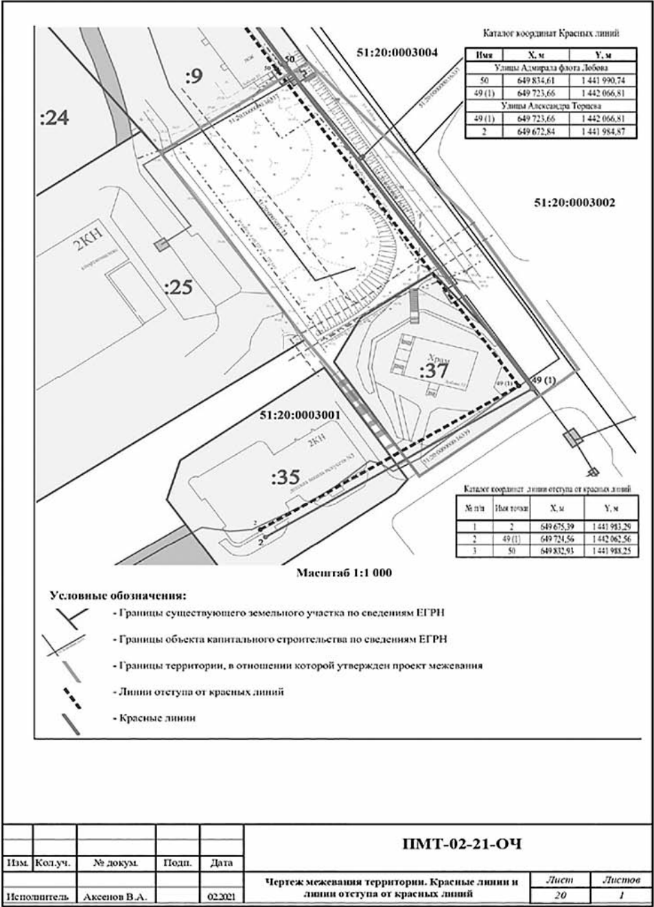
2.2. Чертеж межевания территории. Красные линии и линии отступа от красных линий
